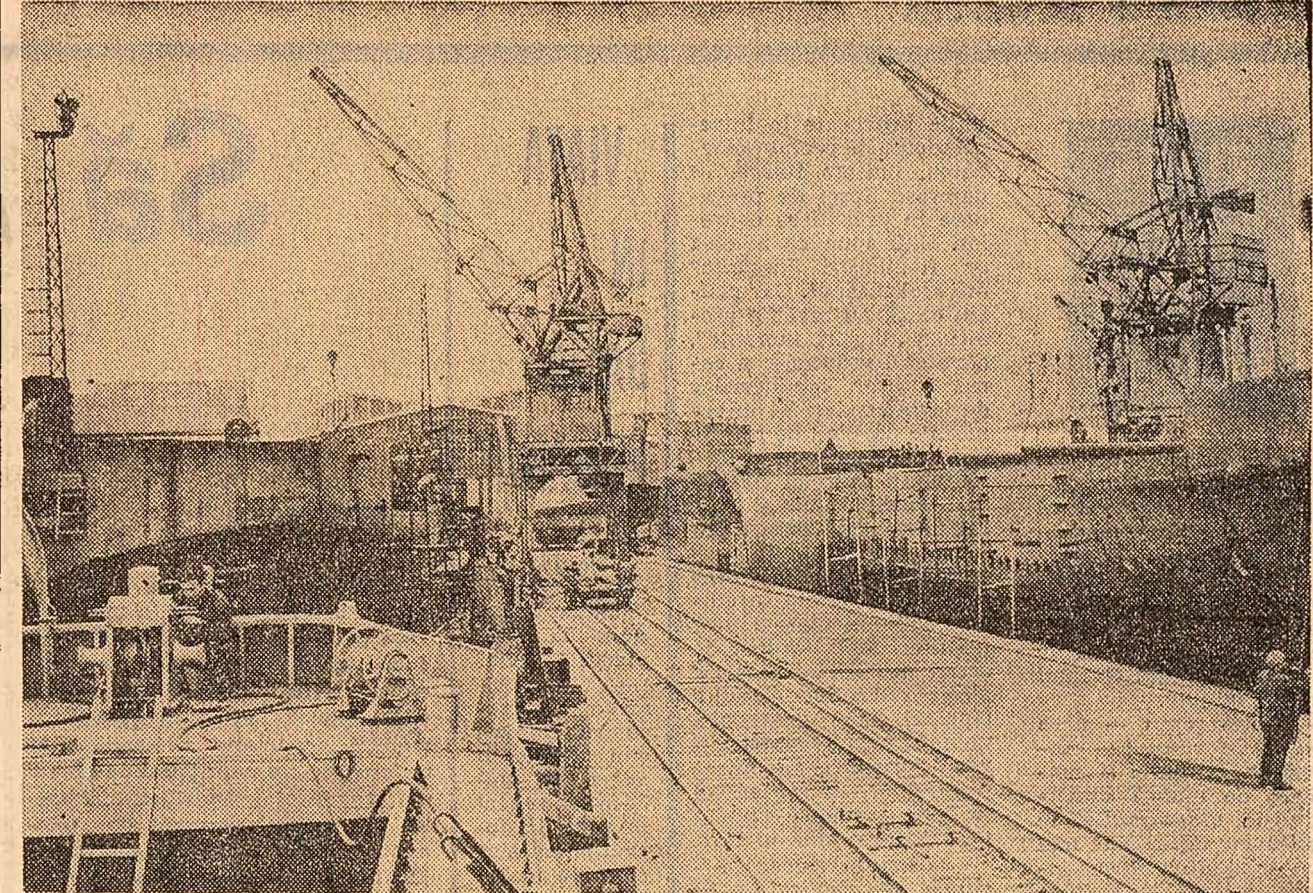
UZINA MECANICĂ DIN TR. SEVERIN: Aspect de pe șantierul de construcție a navelor (Foto: Agerpres)
