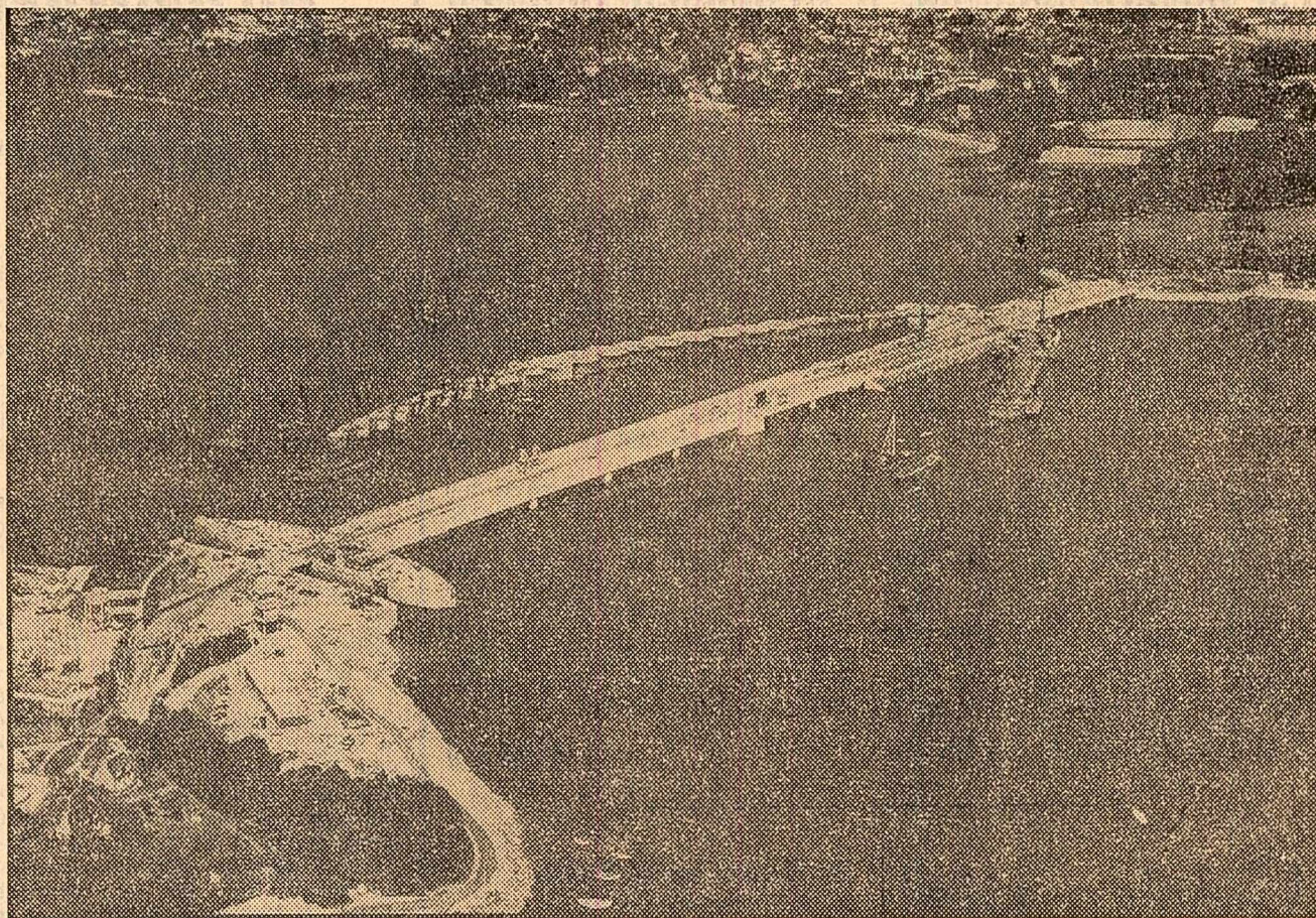
Prima instalație din lume care folosește mișcarea marelui mare pentru a produce energie electrică — uzina marematrice de pe fluviul Rance — a fost inaugurată sâmbătă de președintele de Gaulle. În vara anului viitor, când uzina va fi definitiv terminată, ea va avea o putere instalată de 240 000 kW și va produce anual 544 000 000 kWh.
