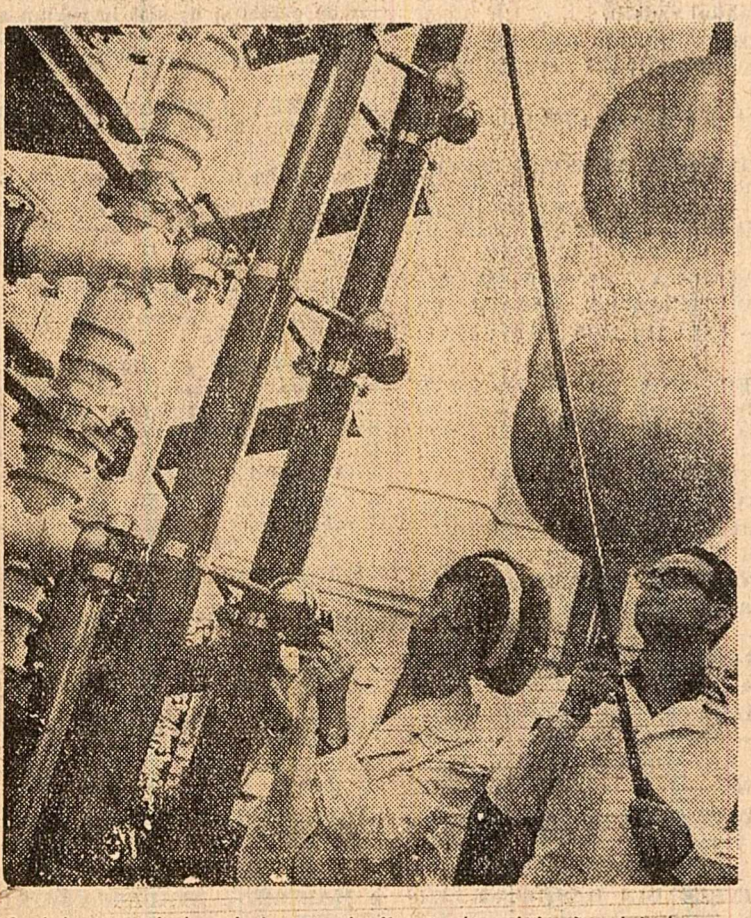
În laboratorul de tehnica tensiunilor înalte al Institutului de cercetări și proiectări electrotehnice București
