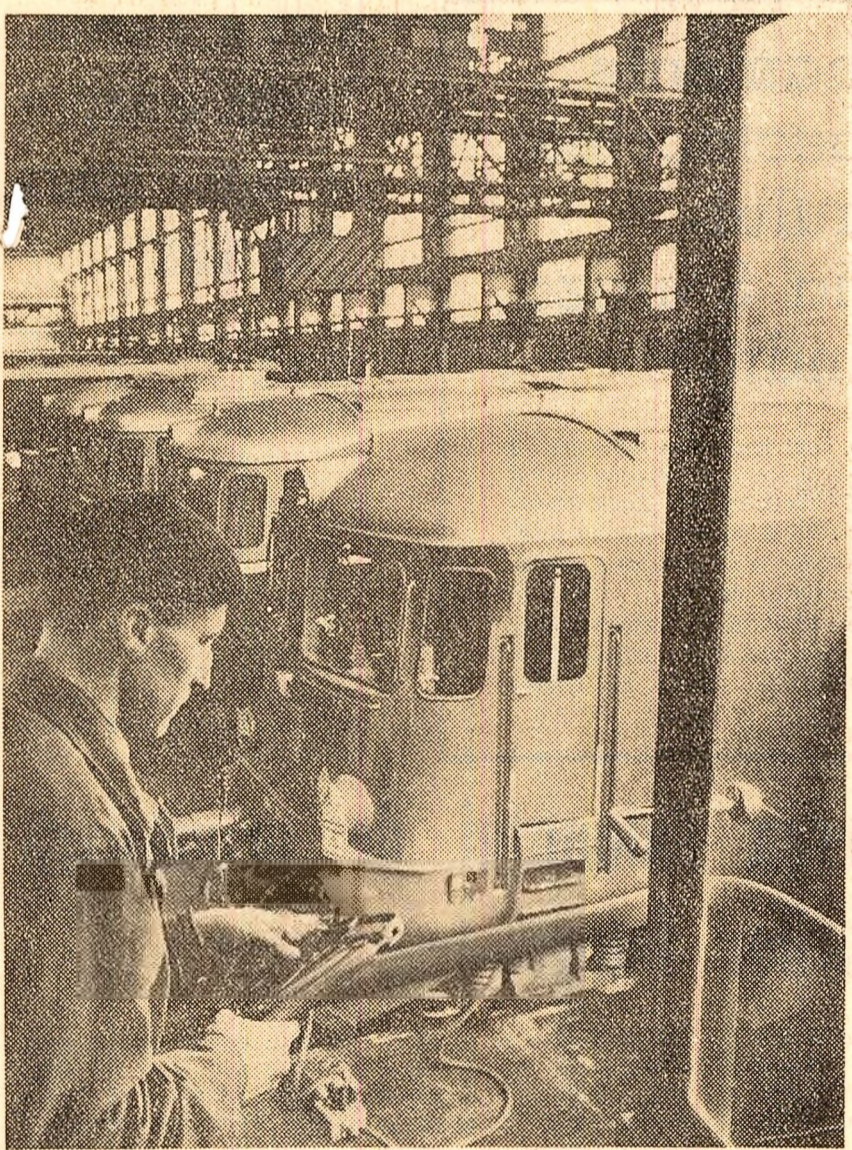
Uzina „Electroputere”-Craiova : noi locomotive Diesel electrice în montaj Foto : M. Andreescu
