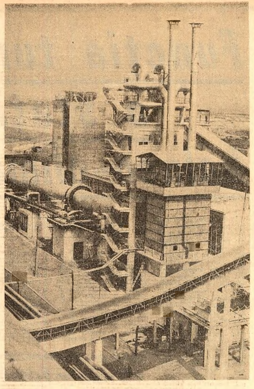
Instalații la Uzina de aluminiu Oradea. Foto: M. Andreesen
