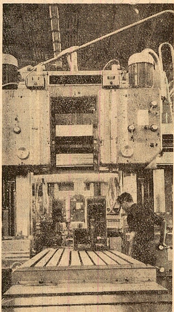
Fabrica de mașini-unelte și agregate — București. Freză portal de 1.000 mm intrată de curînd în fabricația de serie
