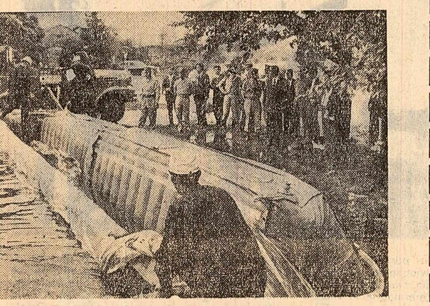
În Japonia se experimentează un nou sistem de stăvîlire a apelor în timpul inundațiilor: se construiesc stăvîlire formate din saci de material plastic umpluți cu apă.
