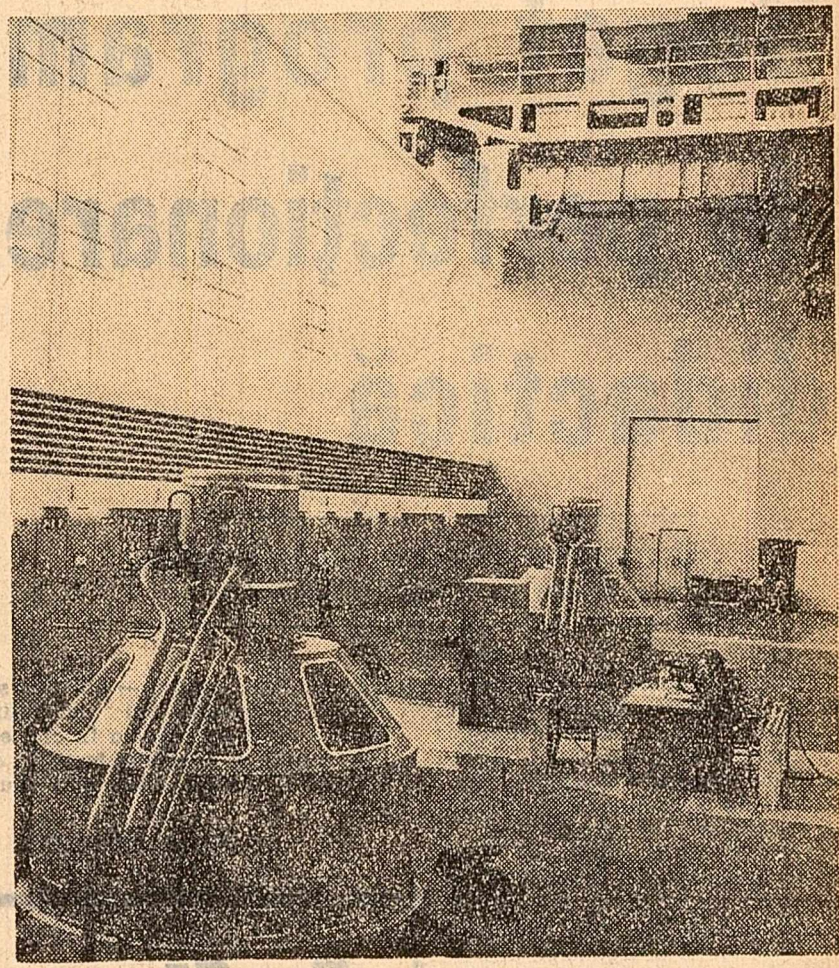
Sala turbinelor de la hidrocentrala Racova de pe Bistrița
