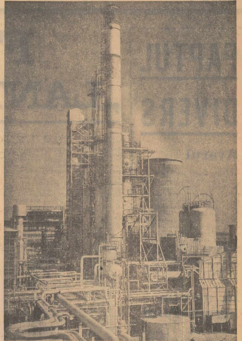
Complexul de cracare catalitică din cadrul Rafinării Brazi, complet automatizat. Foto: Gh. Vințiliă
