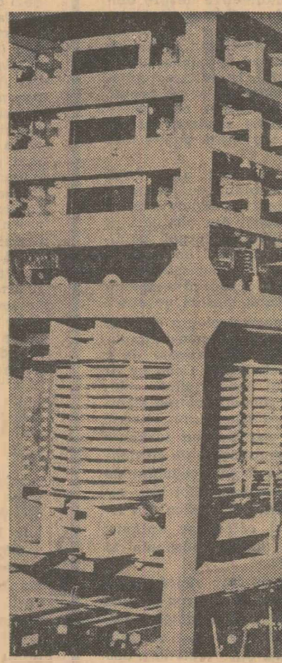
Marca întreprinderii „Electrotehnica”-București a fost aplicată recent pe un nou produs: instalația de redresare pentru asperizarea foililor de aluminiu (în fotografie). Ea este folosită de Fabrica de piese radio și semiconductoare Băneasa la realizarea condensatorilor electrolitici. Instalația realizată în țară are un nivel tehnic superior celor existente, aduse din import, asigurînd îmbunătățirea calității produselor și creșterea productivității muncii
