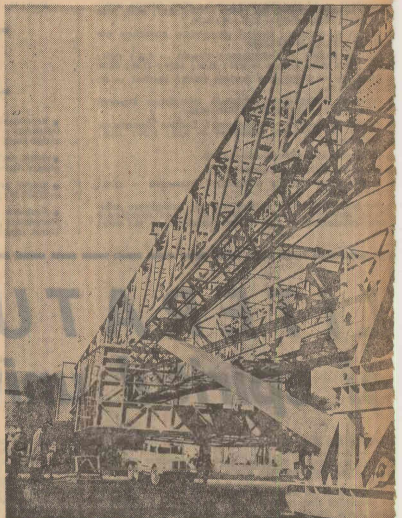
Uzinele „1 Mai”-Ploiești. Instalația 3DH-250 pentru foraj de mare adîncime pe bancul de roci. Foto: Agerpres
