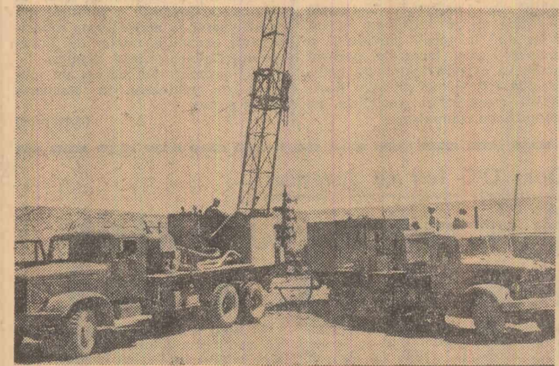
Lucrări de forare pentru prospectarea de noi zăcăminte de petrol și gaze în Afganistan
