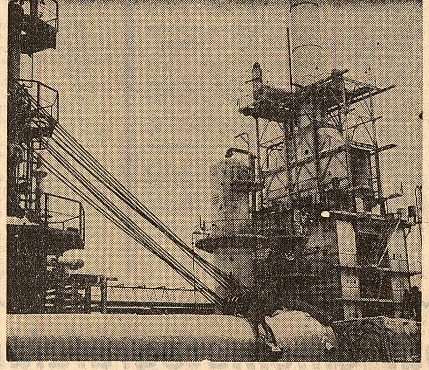
Combinatul de îngrășăminte azotoase Tg. Mureș, Cuptorul de cracare catalitică al noii fabrici de amoniac, în construcție, în etapa a II-a de dezvoltare. Foto: A. Carțean
