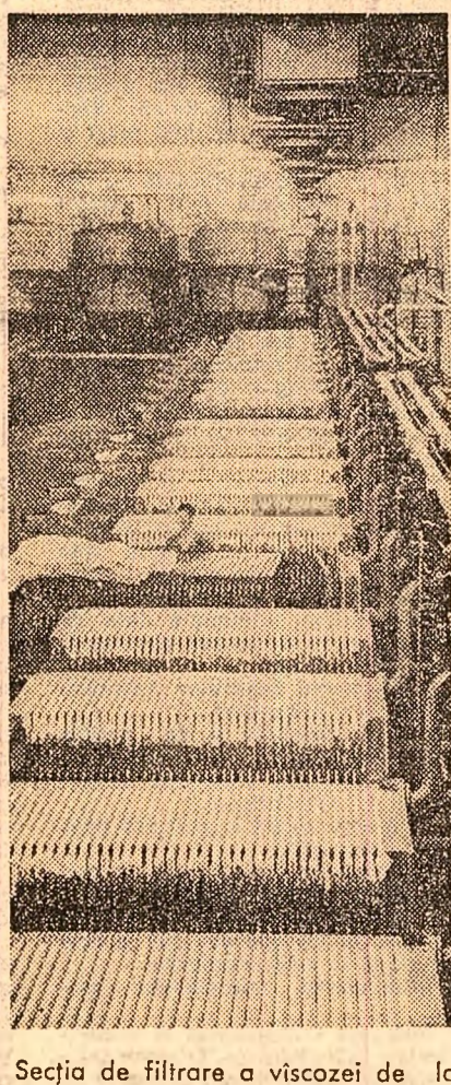
Secția de filtrare a viscozei de la Combinatul de fibre artificiale Brăilă
