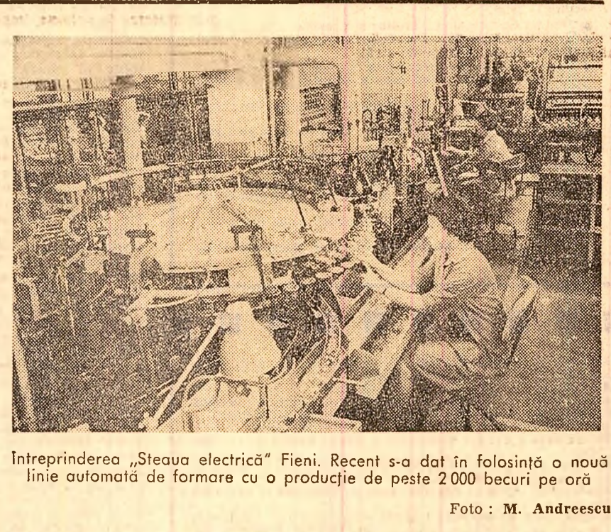
Întreprinderea „Steaua electrică” Fieni. Recent s-a dat în folosință o nouă linie automată de formare cu o producție de peste 20 000 bucuri pe oră
