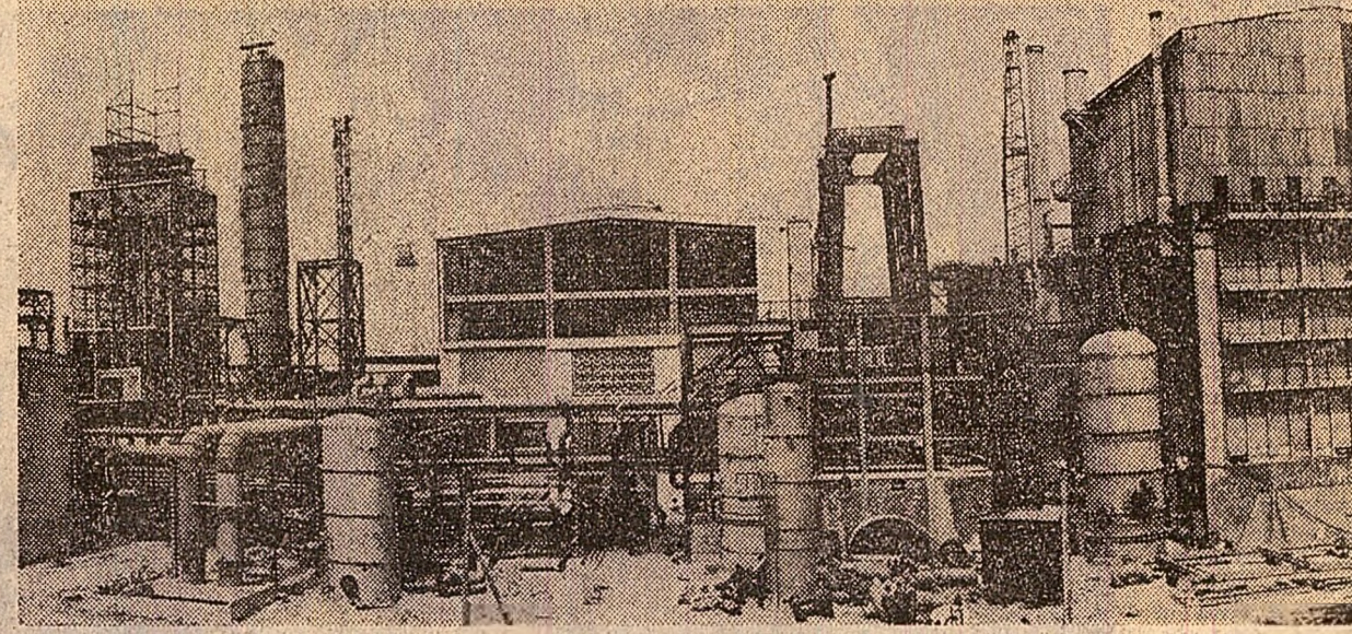
Pe șantierul unității de îngrășăminte azotoase de mare capacitate nr. 1 din Craiova Foto: Gh. Vintilă
