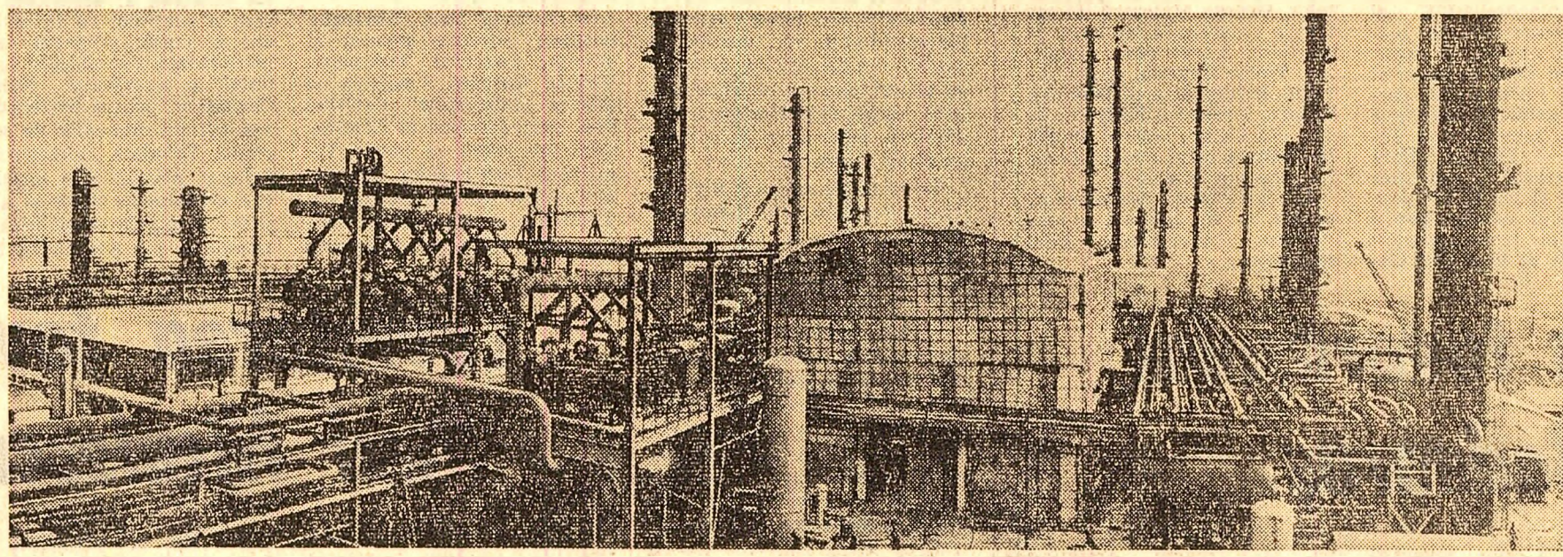
Combinatul petrochimic din Pitești: instalația de piroliză a benzinei - una din instalațiile de mare randament, care asigură valorificarea superioară a materiei prime (Foto: Gh. Vințilă)
