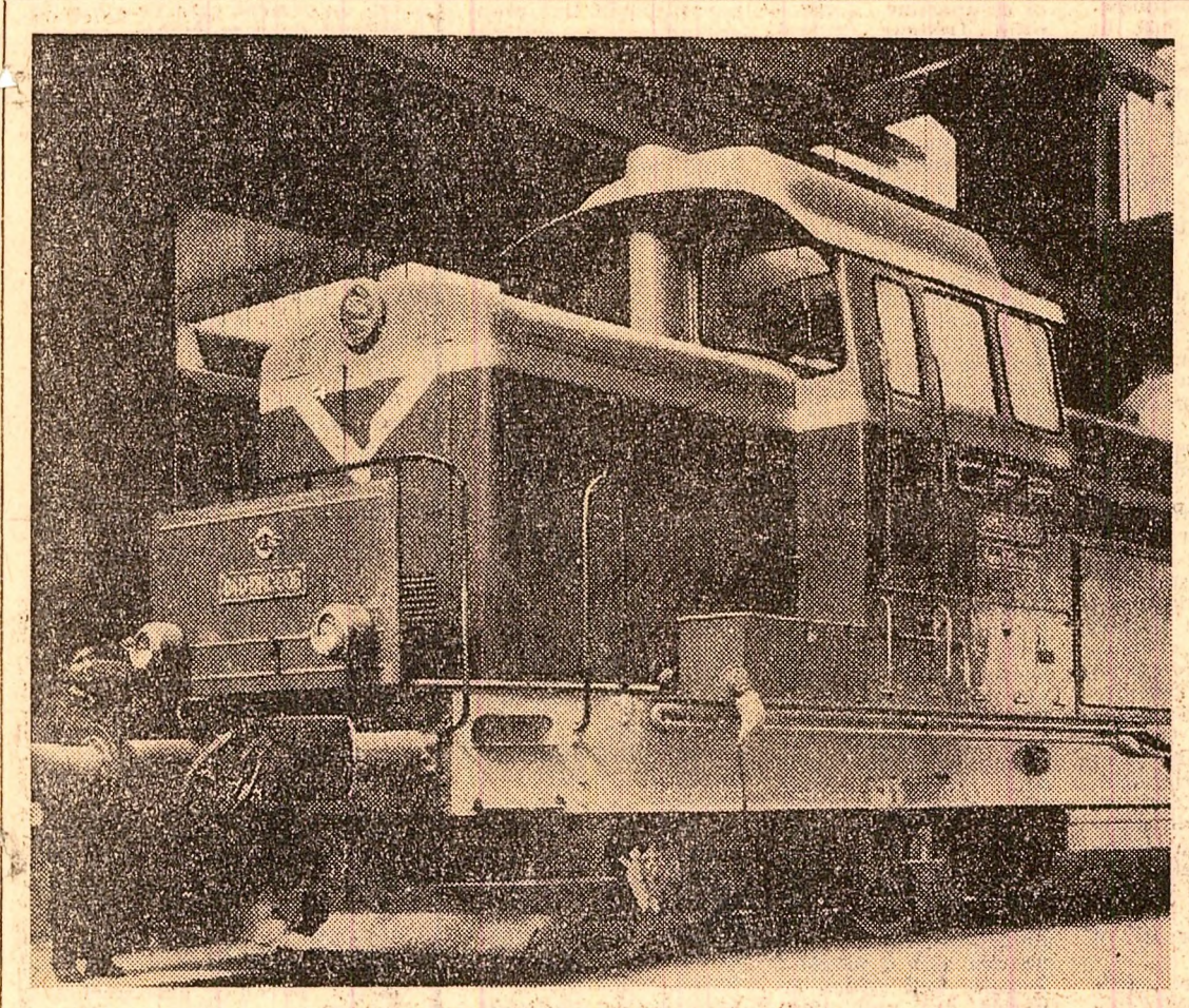
Uzinele „23 August” din Capitală. O nouă locomotivă Diesel-hidraulică de 1250 C.P. Foto: M. Cioe
