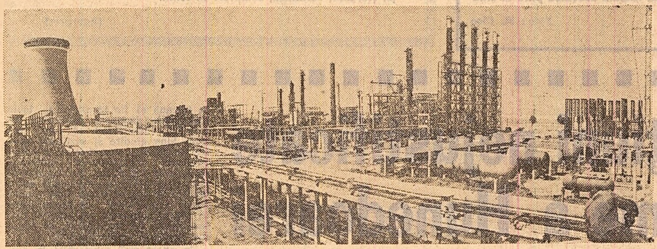
Conducte și coloane pe șantierul Rafinării din Pitești. Foto: Gh. Vințilă
