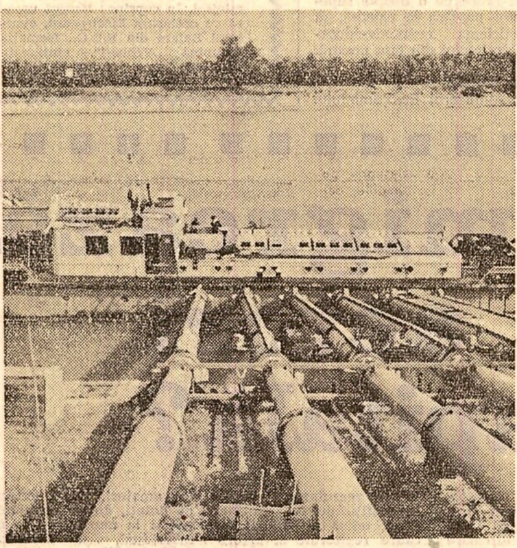
Stația de pompare Modelu, din sistemul Terasa Căldrași asigură apa necesară pentru irigația a aproximativ 10.000 hectare
