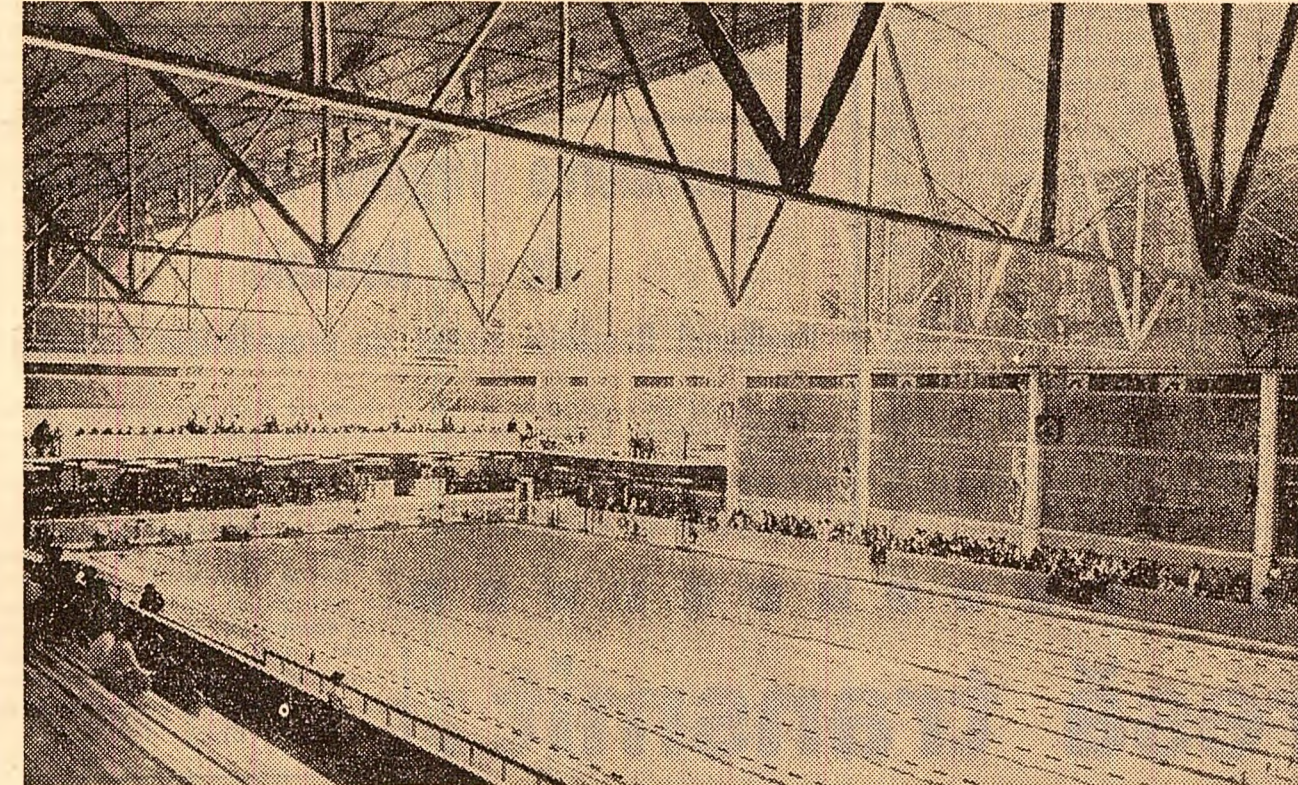
Piscina de la Ciudad de Mexico care va găzdui întrecerile olimpice de natație. Partea centrală a acoperisului este făcută dintr-un material translucid. Într-un bazin alăturat se vor desfășura probele de sărituri de pe trambuline.
