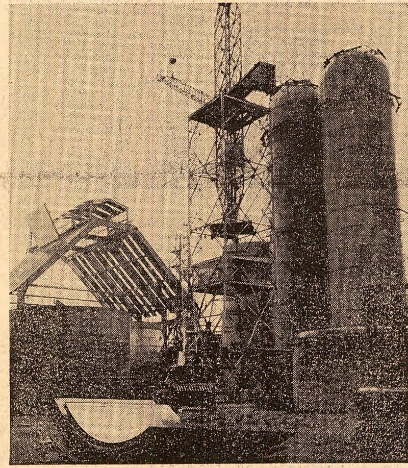
Combinatul siderurgic „Gh. Gheorghiu-Dej” din Galați. Imagine de pe șantierul furnalului numărul 2 de 1700 mc., aflat în construcție (Foto: Gh. Vințilă)
