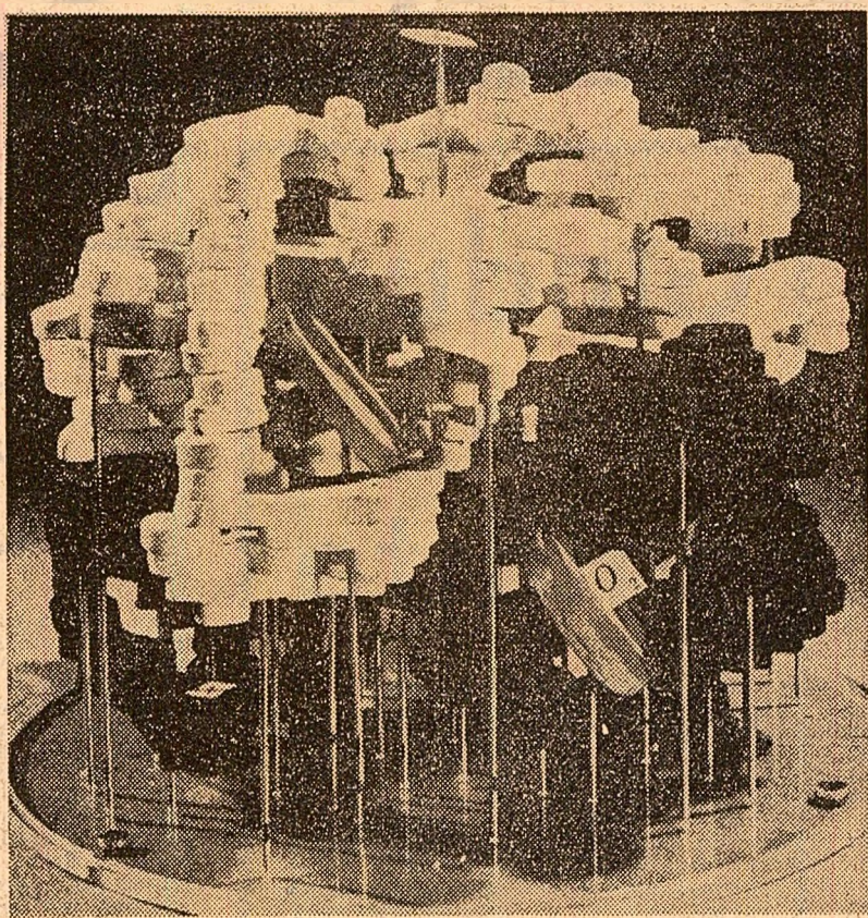
Modelul moleculei de hemoglobină dedus în urma studiilor efectuate prin difracția razelor X
