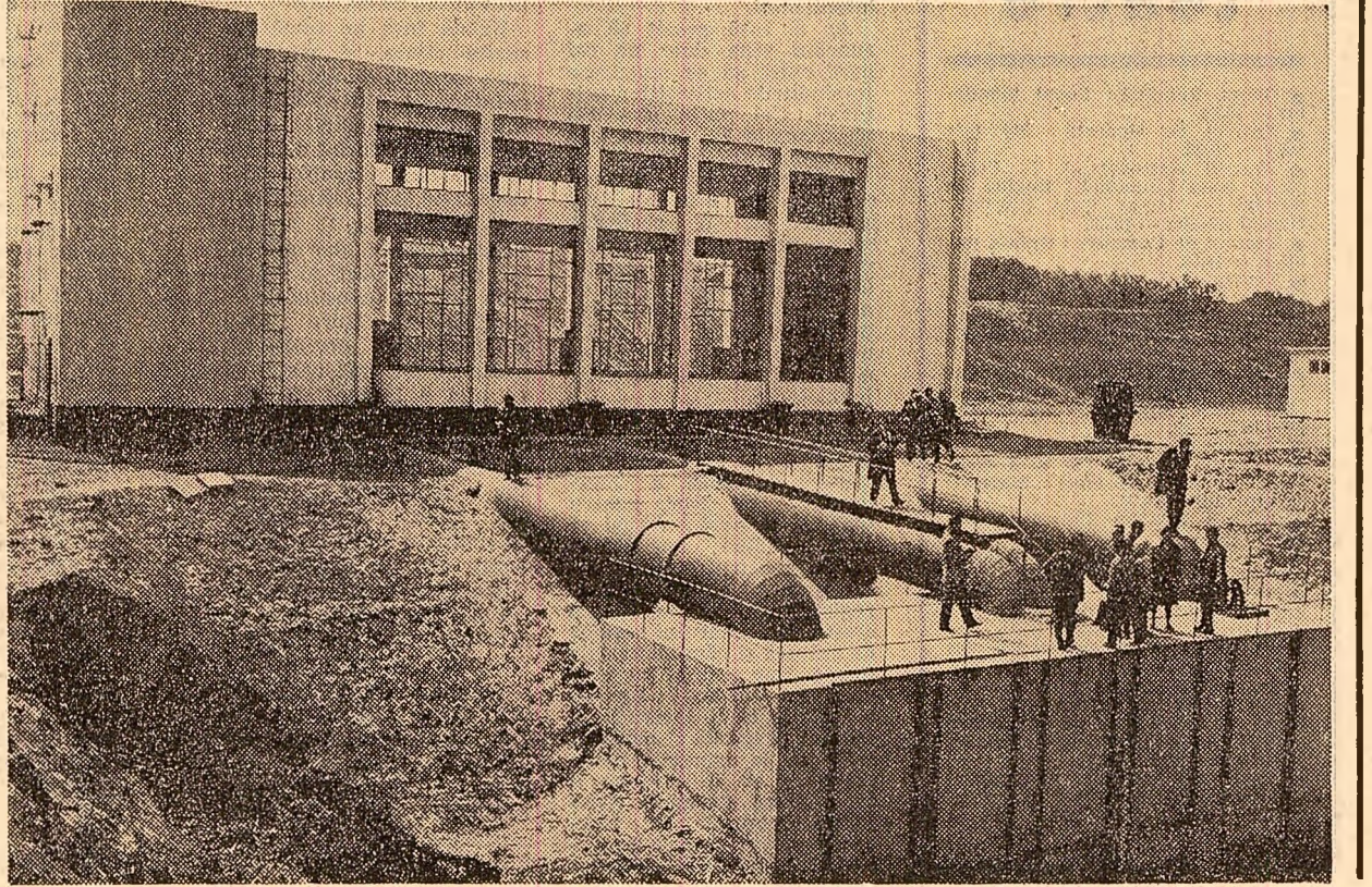
Stația de pompare de la I.A.S. Greaca, județul Ilfov Foto: M. Andreescu
