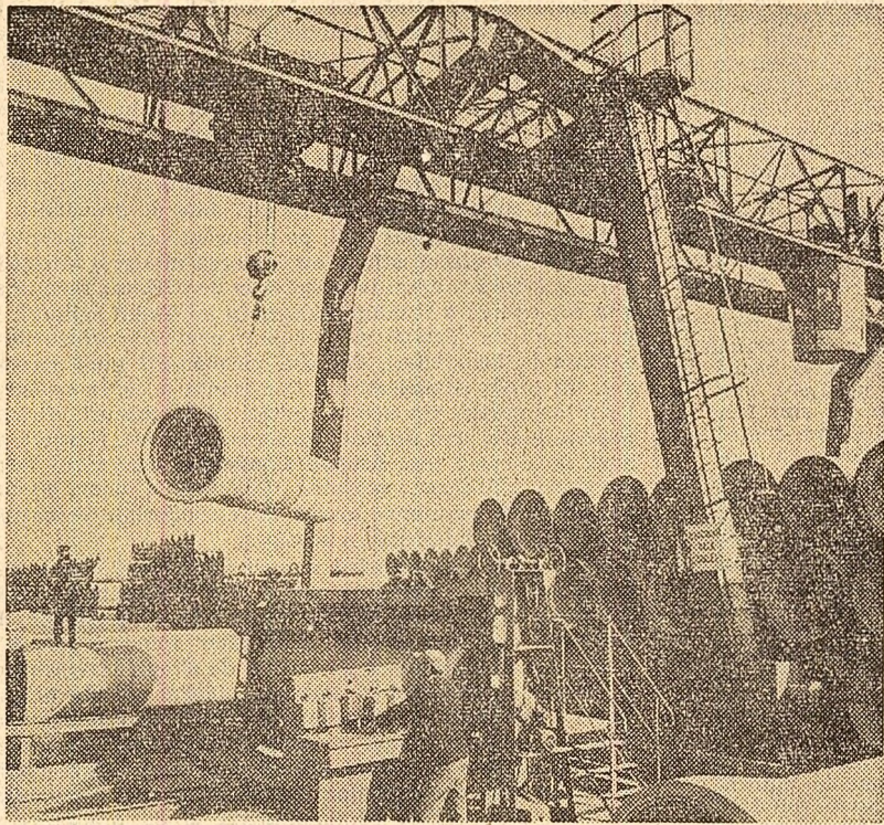
La întreprinderea „Progresul” din Capitală se realizează un sortiment variat de prefabricate din beton, beton precomprimat și armat destinat construcțiilor industriale și de locuințe. În fotografie: instalația de aplicare a stratului de protecție la tuburile din beton precomprimat prin vibrolaninare, o invenție românească aplicată în întreprindere. (Foto: Agerpres)
