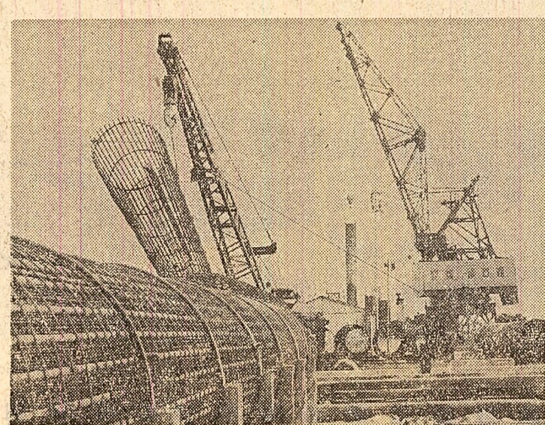
Pe șantierea podului de peste Dunăre, Giurgeni—Vodul Oii Foto: A. Cartojan
