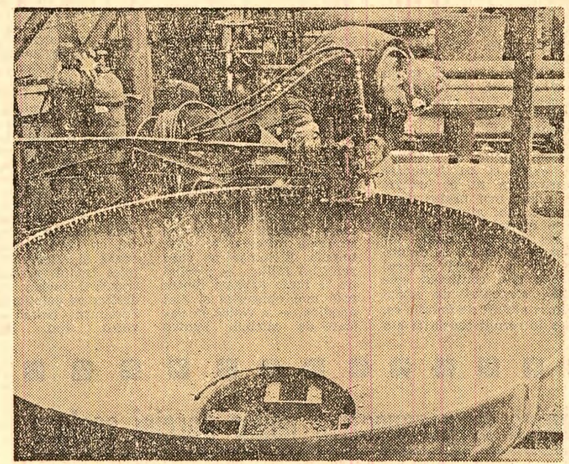
Echipament tehnologic în execuție la Uzina de utilaj chimic din Capitală. Foto: Agerpres
