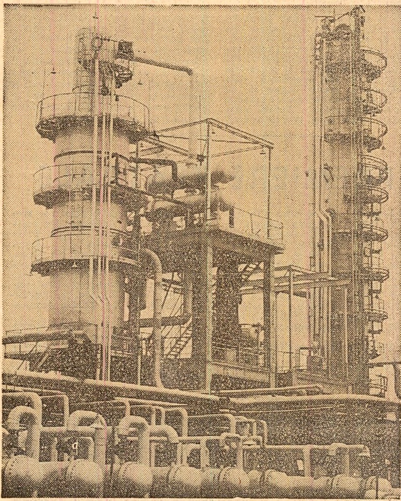
Instalații ale noii rafinării „Crisana” din Suplacu de Barcău, județul Bihor, cu o capacitate de prelucrare de 300 000 tone țîței pe an (Foto: Gh. Vințu)
