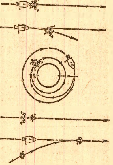
Schema programului autonom de zbor al modulului lunar
