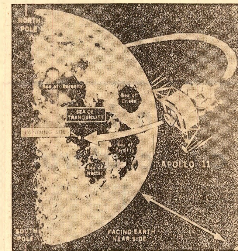
Schema traiectoriei modulului spre Lună. Săgeata indică regiunea de contact cu suprafața lunară. (Fotografia de sus) Așa arată locul aselenizării. (Fotografia de jos)
