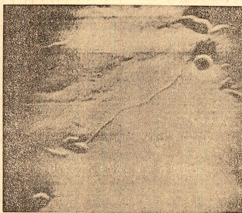
Schema traiectoriei modulului spre Lună. Săgeata indică regiunea de contact cu suprafața lunară. (Fotografia de sus) Așa arată locul aselenizării. (Fotografia de jos)
