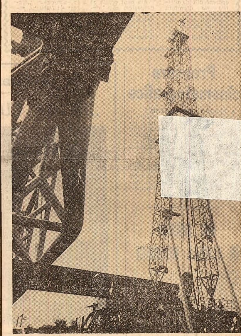
Tipuri din cele mai moderne sonde: F 200-2 DH și ultima creație, F 125-2 DH tip nou, realizări ale constructorilor de la uzina „1 Mai” Ploiești. Foto: M. Andreescu
