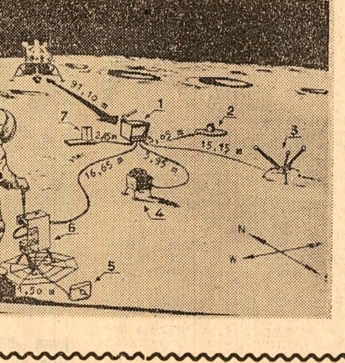
Schema „Alep”-ului: 1. post central; 2. seismograf; 3. magnetometru; 4. spectrometru; 5. detector catodic pentru măsurarea atmosferei; 6. detector surtermic de ioni; 7. generator. (fotografia din dreapta)
