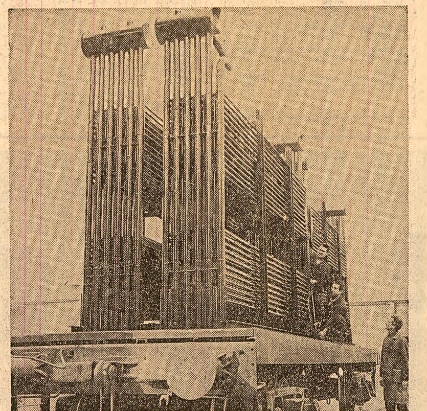
Renumele uzinei „Vulcan” din Capitală a depășit cu mult hotarele țării, produsele sale fiind deosebit de apreciate de firme industriale de prestigiu din numeroase țări. Imaginea de mai sus reprezintă ansamblu ale unui cazan de 50 G/cal destinat exportului
