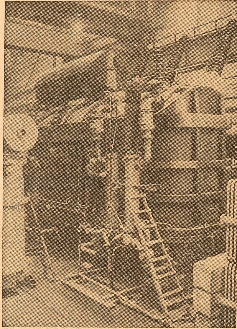
Prima transformator electric de 190 MVA, realizat la uzina „Electroputer” din Craiova (în fotografie). Soluțiile adoptate la construcția lui sînt în întregime originale și aparțin specialiștilor craioveni. Noul transformator, destinat echipării centralei hidroelectrice de la Porțile de Fier, are parametrii funcționali asemănători cu cei realizați de firme bine cunoscute din diferite țări dezvoltate din punct de vedere industrial. Foto: M. Andreescu
