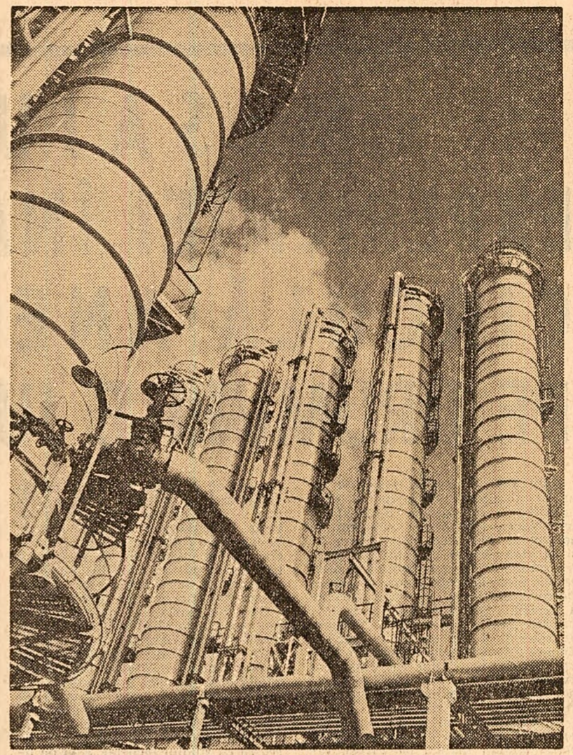
Imagine de la instalația de xilen din cadrul Rafinării Brazi. Foto: Gh. Vințila
