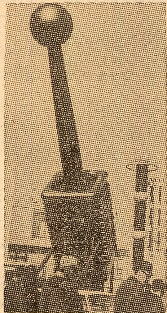
Această instalație uitașă, realizată pe baza unui nou sistem de construcție, servește la verificarea izolațiilor, conductelor și aparatelor electrice cu o tensiune pînă la 1200 kilovolți. Sistemul hidrolic de glisare, acționat cu mijloace proprii, permite intrarea în funcțiune fără o montare prealabilă. Instalația a fost produsă de Uzina de transformatoare și aparate Röntgen din Dresda (R.D.G.).
