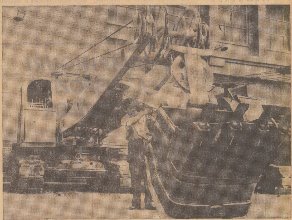
Uzina de utiloj greu din Brăila: noul tip de excavator de 0,6 mc aflat în probe finale
