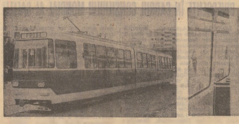
Fotografia de mai sus vă prezintă prototipul noului vagon de tramvai silențios V3A-I.T.B. realizat de către colectivul de muncitori, tehnicieni și ingineri de la Întreprinderea de transport București. Caracteristicile sale se înscriu la
