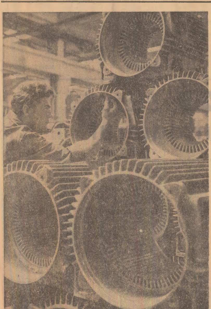
Uzina de mașini electrice din Capitală. Un nou lot de staționare poate intra în montaj. Foto: Agerpres
