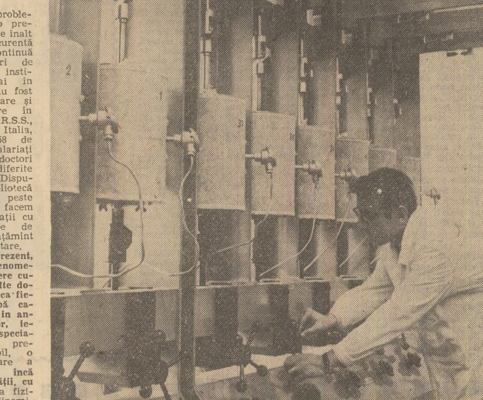
Laborator pentru încercarea oțelului la flux din cadrul Institutului de cercetări metalurgice
