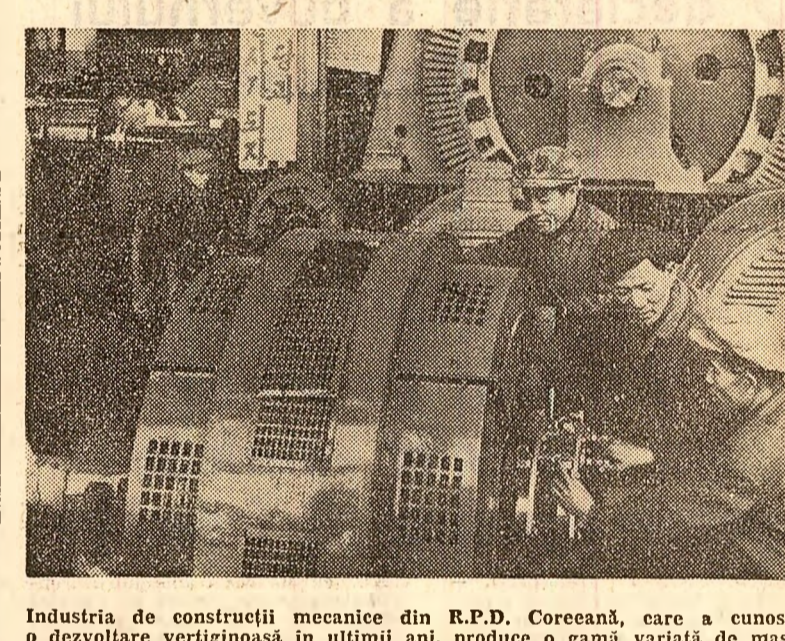
Industria de construcții mecanice din R.P.D. Coreeană, care a cunoscut o dezvoltare vertiginosă în ultimii ani, produce o gamă variată de mașini și echipamente, mașini-unelte de mare capacitate, prese de mai multe mii de tone, transformatoare de înaltă tensiune, motoare Diesel, excavatoare, tractoare, camioane. În prezent, această industrie furnizează economiei naționale nord-coreene toate mașinile și echipamentele, de la cele mai simple, pînă la cele mai complexe și de înaltă precizie. În imagine s-a înregistrat atelierul de fabricație ale întreprinderii de utilaj energetic Ceilima Taen
