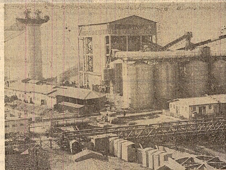
Complexul de betoane de la Porțile de Fier Foto: Gh. Vințilă
