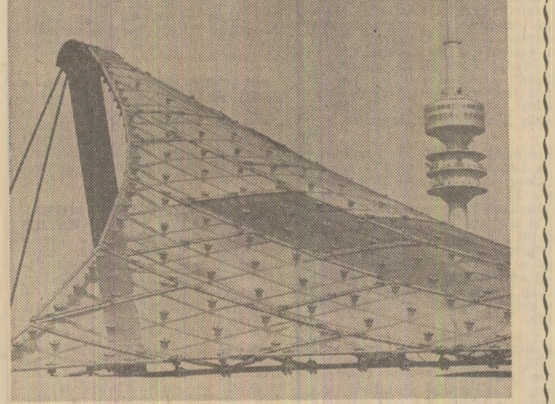
Vedere parțială a acoperisului Stadionului Olimpic din München. În planul al doilea: turnul de televiziune, înalt de 220 metri
