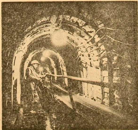
Banda transportoare de cărbuni de la mina Paroșeni Foto: N. Moldoveanu
