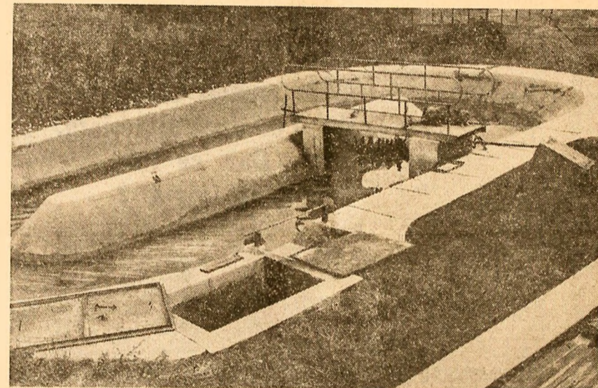
În stațiile pilot de epurare pot fi experimentate și omologate diferite instalații de epurare a apelor uzate care provin de la orașe și industrii. (În fotografie: șanțul de oxidare totală în curs de omologare la Institutul de studii, cercetări și proiectări pentru gospodărirea apelor (I.S.C.P.G.A.)
