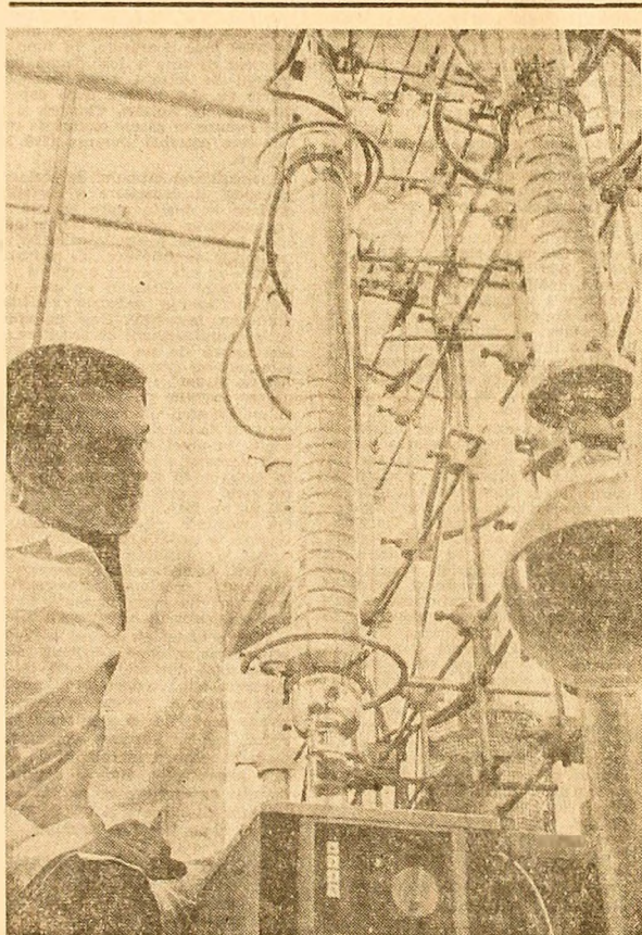
Căuțind să răspundă cât mai prompt problemelor de producție, laboratorul de polimerizări de la Combinatul petrochimic Pitești efectuează cercetări pentru obținerea unor noi sortimente de mase plastice. În fotografie: inginerul cercetărilor, Bader Berard Lucind la o coloană de distilare pentru purificarea monomerilor
