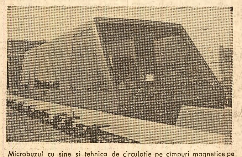
Microbuzul cu șine și tehnica de circulație pe cîmpuri magnetice pe linia experimentală Ottobrunn, lângă München.
