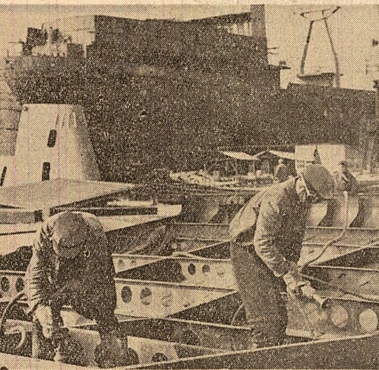
Pe calea de montaj a șantierului naval Turnu Severin
