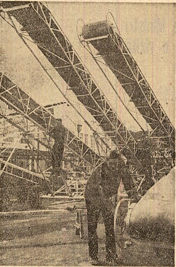
Uzina „Unio” Satu-Mare. Se fac ultimele verificări la un nou lot de transportoare gata de livrare către beneficiar
