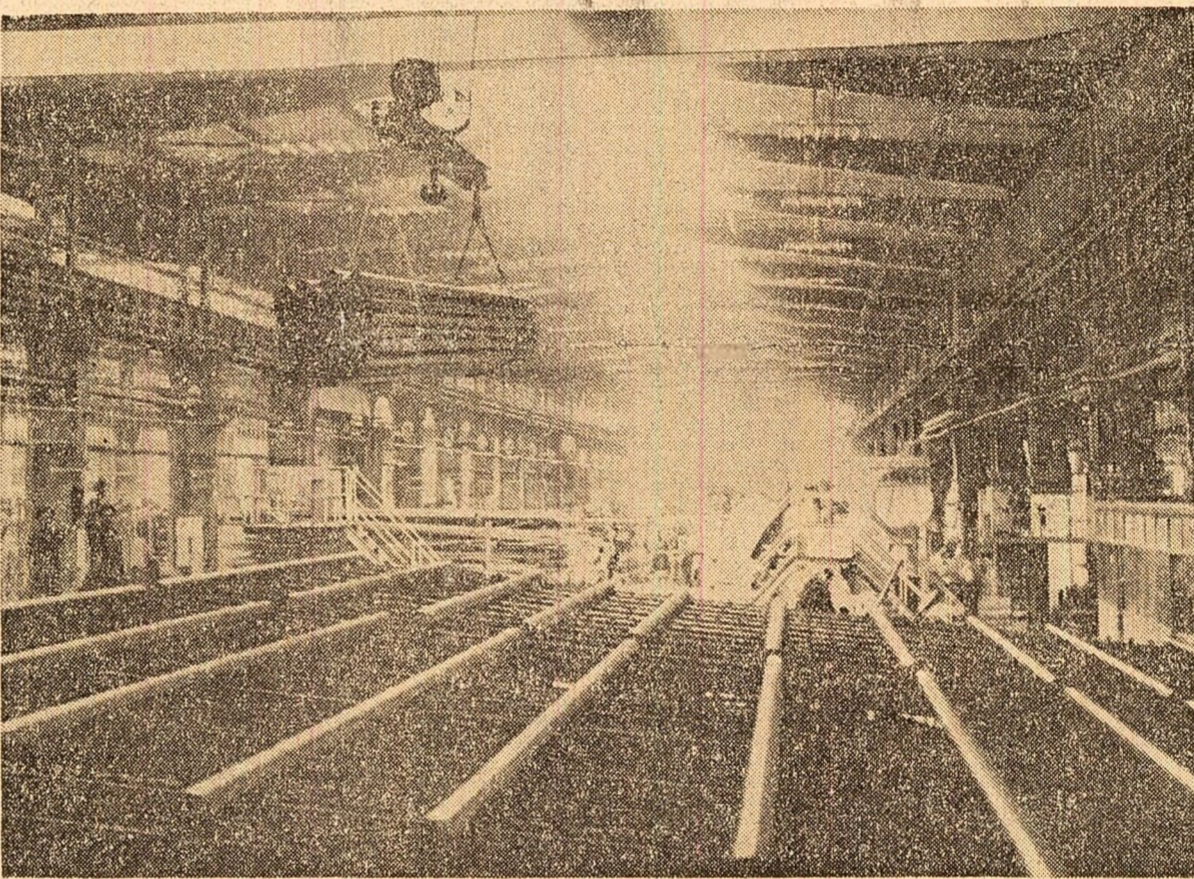
Aici, la Iași, în hale moderne de producție, dotate cu utilaje și tehnologii de înalt nivel tehnic, se produc țevi de diverse dimensiuni necesare economiei naționale. În fotografie: aspect de la Uzina metalurgică
