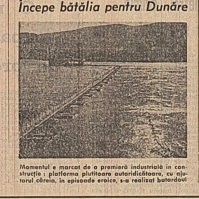
Începe bătălia pentru Dunăre... Momentul e marcat de o premieră industrială în construcție: platforma plutitoare autoriducătoare, cu ajutorul căreia, în episoade eroice, s-a realizat batardoul
