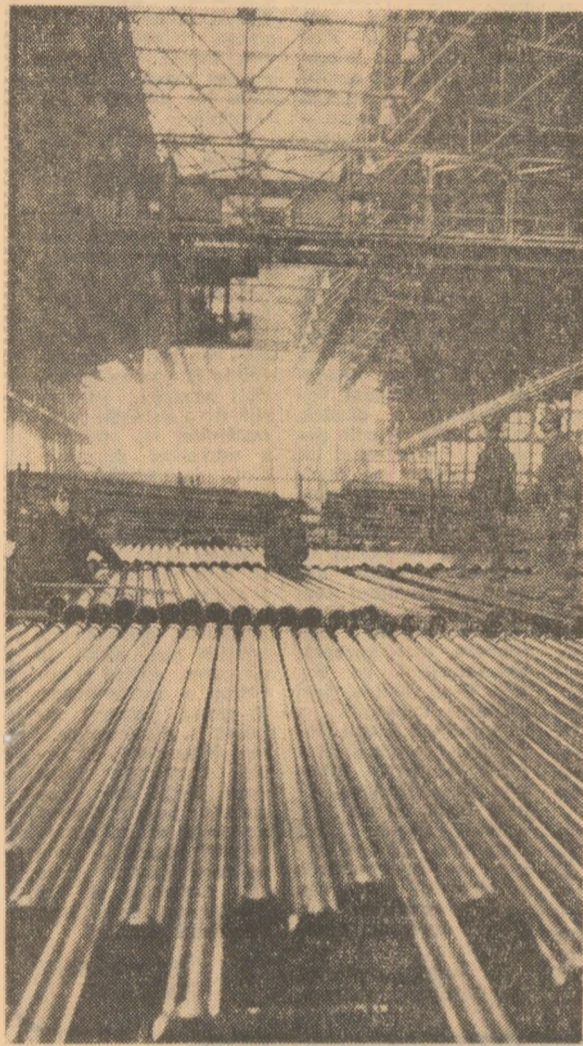
Preocuparea principală a colectivului de muncă de la uzina „Republica” din Capitală este de a obține țevi de calitate 1 în proporție de 95 la sută, precum și asimilarea de produse noi a căror valorificare aduce un mare venit uzinei. Se depun, de asemenea, eforturi pentru reducerea consumului specific de otel, unde s-a ajuns la o medie de 2 kg per tonă
