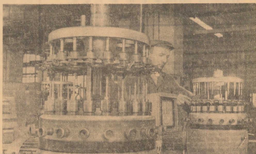
Tehnică modernă, hărnicia și inițiativa creatoare — iată izvoarele succeselor de prestigiu obținute până în prezent de colectivul Uzinei de mecanică fină din Sinaia, în îndeplinirea planului și angajamentelor. În fotografie: un exponat al acestei tehnici — mașina de lepuț cu 20 de posturi de lucru, deservită de un singur muncitor, realizată în uzină, prin autofiliere
