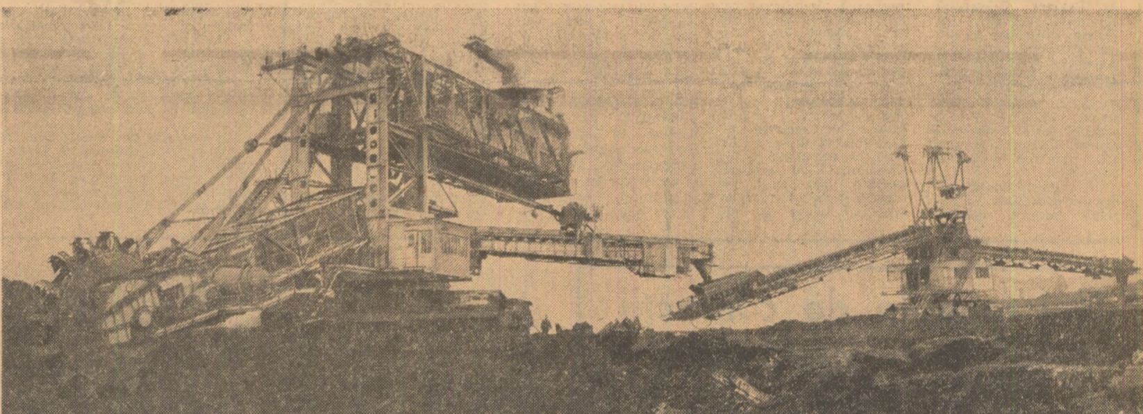
Exploatarea minieră la zi — Căminul din bazinul carbonifer Rovinari, de unde prezentăm această fotografie, dispune de mașini și utilaje care asigură un înalt grad de mecanizare a lucrărilor. Folosind cu pricepere tehnica modernă din dotare, colectivul său de muncă a obținut peste plan, în 11 luni din acest an, 212 000 tone cărbune Foto: S. Cristian
