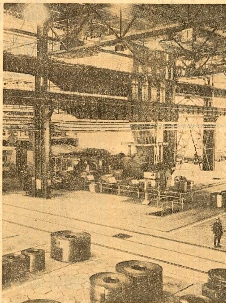
Înaltul grad de tehnicitate al instalațiilor aflate în dotarea Combinatului siderurgic din Galați asigură realizarea unor produse de bună calitate, intens solicitate de beneficiarii interni și externi. În imagine: secția tandem a laminorului de benzi la rece din cadrul combinatului. Foto: E. Dichisceanu
